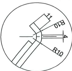
Detalj - A
